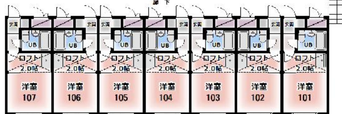
【1階平面図】
